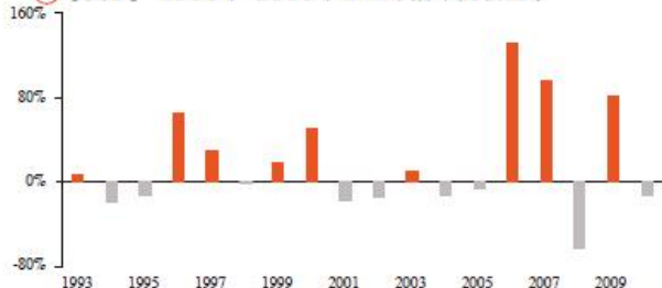
【图1】 1993年-2010年上证综指年度收益率
