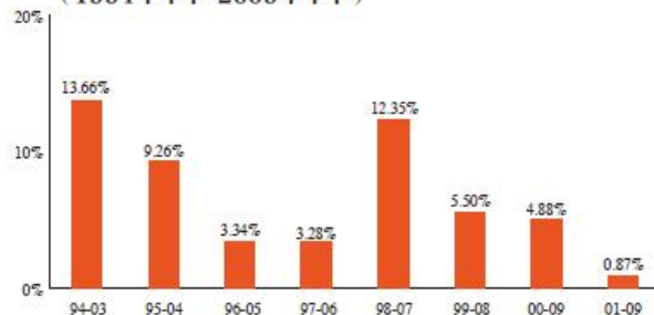
【图3】 中国市场以9年为周期的投资收益情况（1994年年中-2009年年中）
