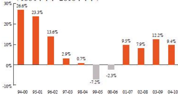
【图2】 中国市场以6年为周期的投资收益情况（1994年年中-2010年年中）
